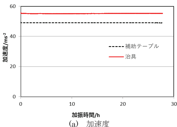
図3 監視信号の経時変化(X方向加振時)
