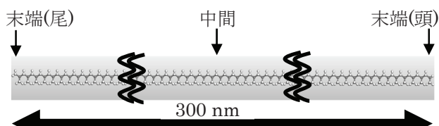
図1 2000量体のPP(アイソタクチック構造)の計算モデル
