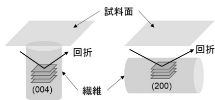
図3 セルロース繊維の試料面に対する方向関係と、回折を生じる結晶面。
