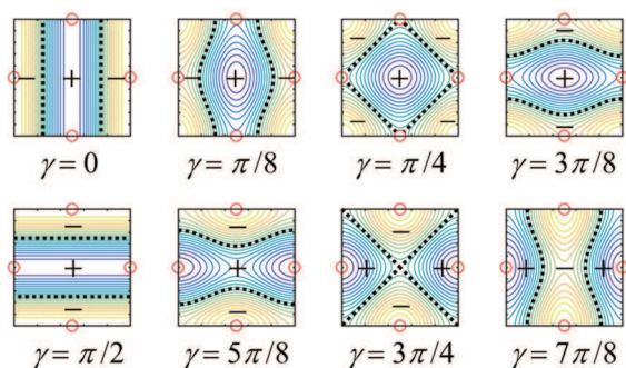
図3 縮退した場合の(2, 0)モード
