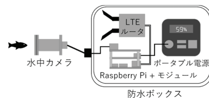
図1 試作したシステムの構成
