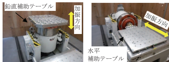
(a)鉛直加振時 (b)水平加振時
