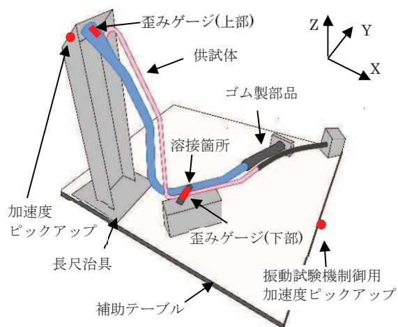
図2 供試体およびセンサの配置図
