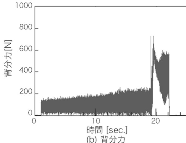
図2 主分力と背分力
