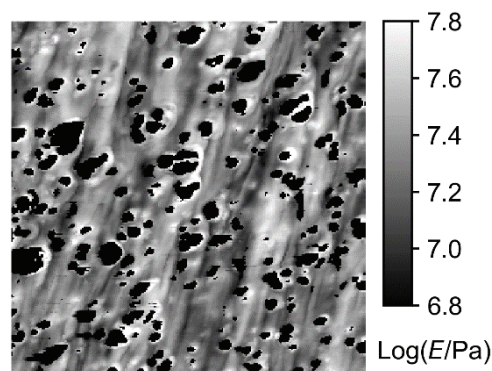
図3 CBを黒色でマスク処理したJKR弾性率像(CB-40の400%伸長)、スキャンサイズは2 μm
