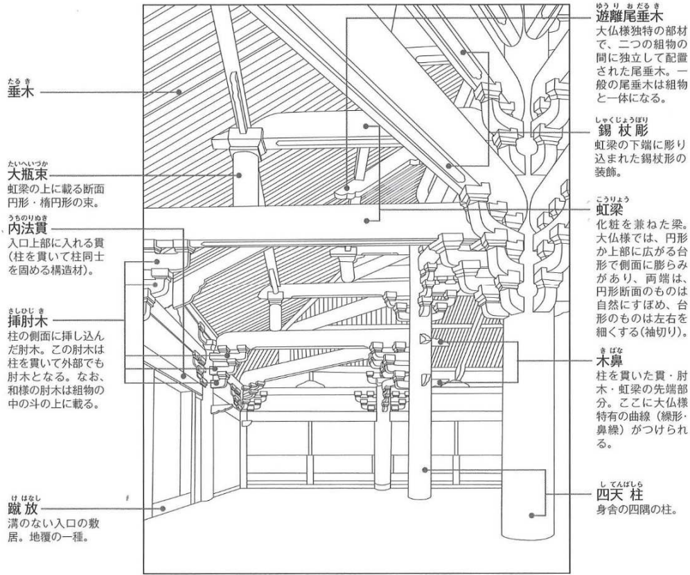
図1 木造建築内部の各部名称 (出典2)
