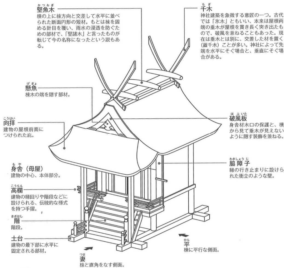
図2 神社の部位名称 (出典2)
