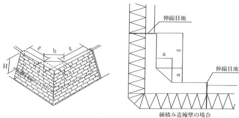
(a) 立体図
