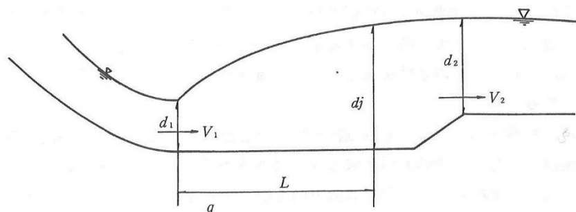
図2 減勢工
