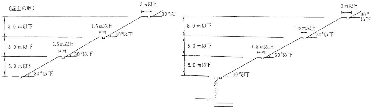
図 盛土の例
