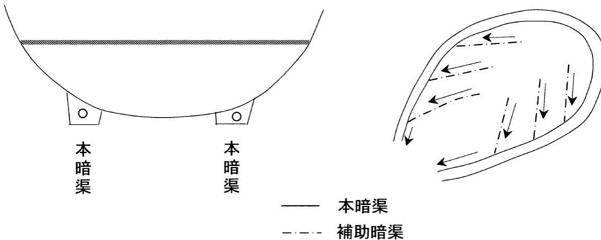
図 遮断式
