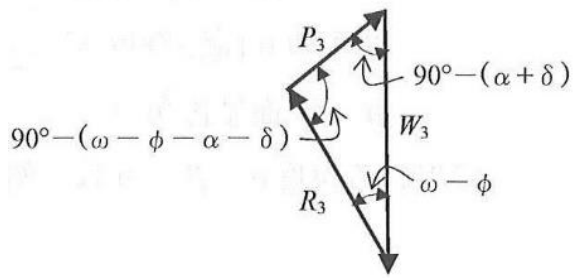
(c) 連力図
