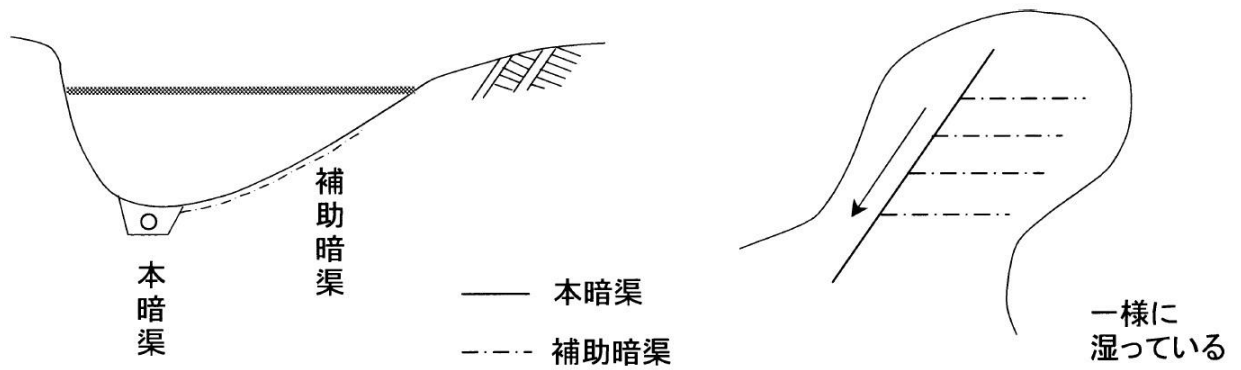
図 くし歯式
