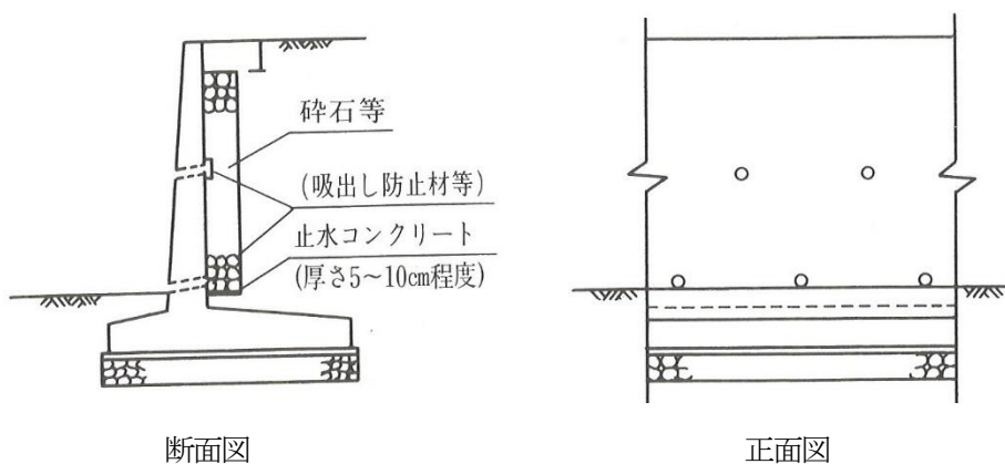
図 水抜穴の配置
