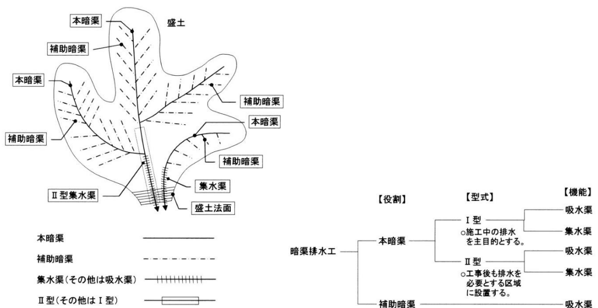
図 地下水排水施設の配置例
