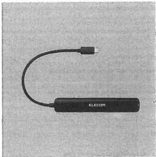
ケーブルは紛失の心配がない直付けタイプです。ケーブルの長さは約17cmです。 ※ USB Type-C™コネクタからの充電に対応しない本体の場合、本製品のUSB Type-C™コネクタ経由での本体充電はできません。充電を行う際は、機器がUSB Power Deliveryに対応していることを確認してください。
