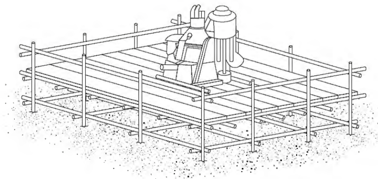
平坦地足場(0.3m 超) (嵩上げ足場)
