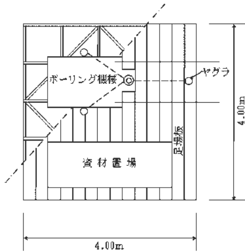
平面図
