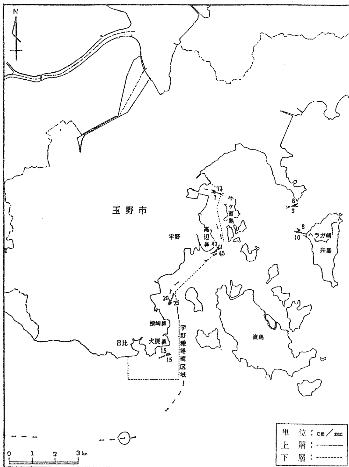
図-9 恒 流 図
