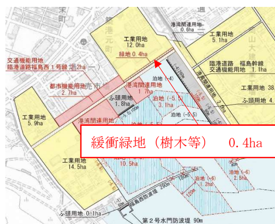
図3-1-1 港湾環境整備施設計画（福島地区）
