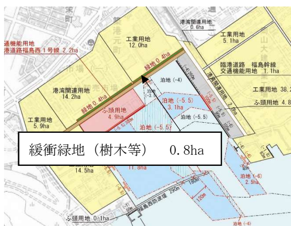
図3-1-1 港湾環境整備施設計画（福島地区）
