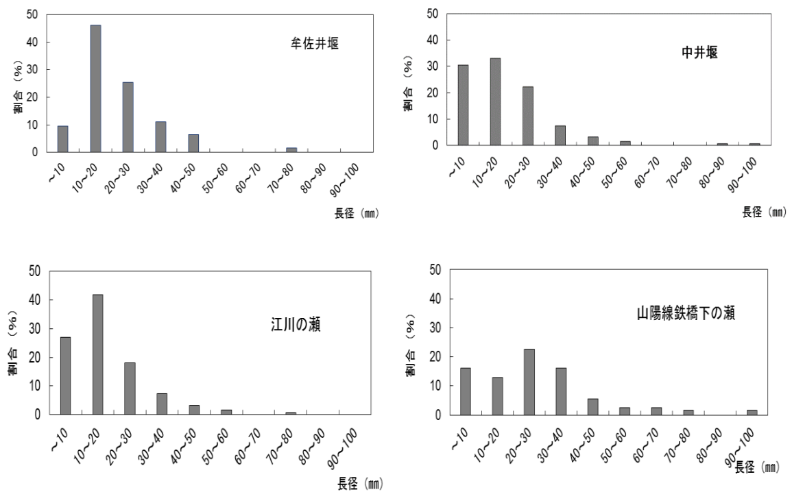
図 7 旭川水系 4 カ所における河床材料の長径組成
