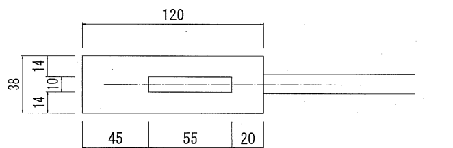
固定金具 頭部詳細図 S=1/1
