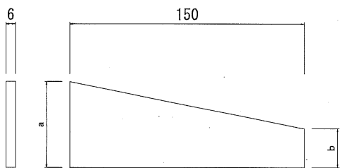
くさび (固定金具用) 一般図 S=1/1
