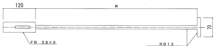
固定金具 一般図 S=1/2
