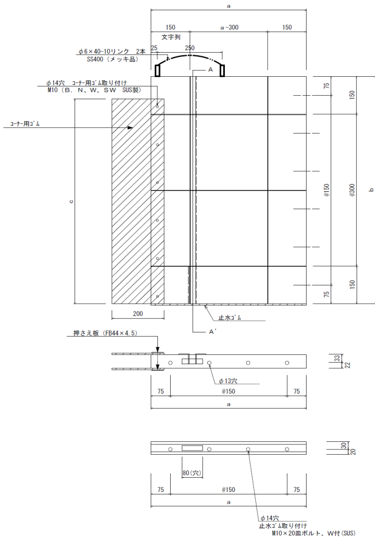
型枠（魚道部） 寸法表
