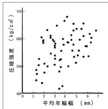
ケヤキ材における平均年輪幅と圧縮強度との関係(橋詰1987)
