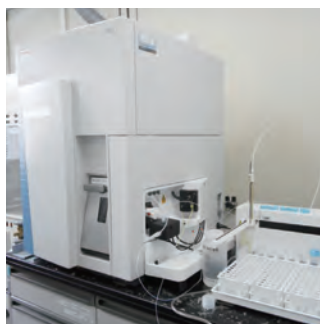
水中のウランを測定する 水中高周波誘導結合プラズマ質量分析装置(ICP-MS)
