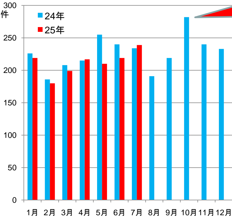
岡山県内の自転車に関連した交通事故(月別件数) 岡山県警交通事故統計より
