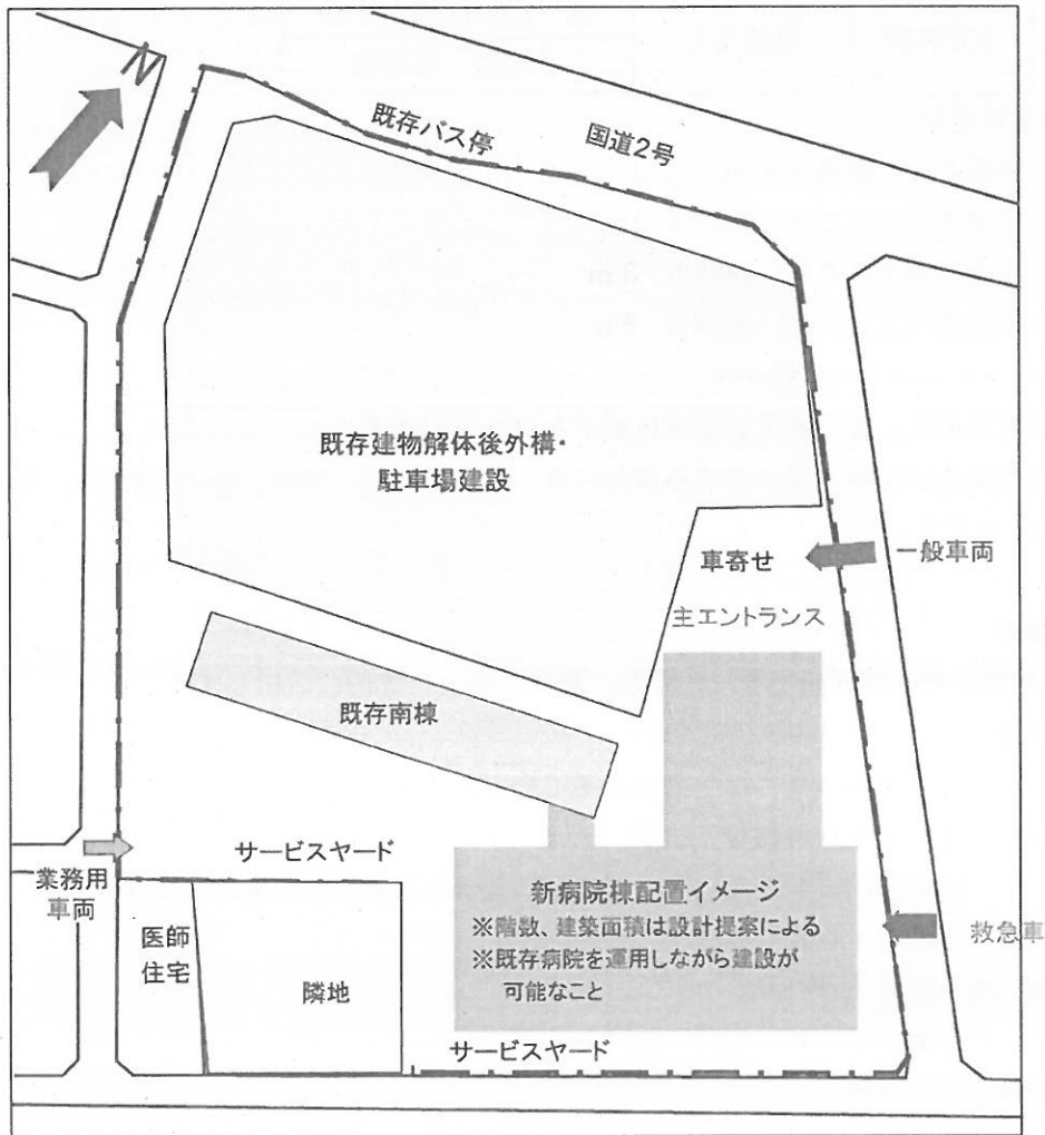
【建物配置計画図】
