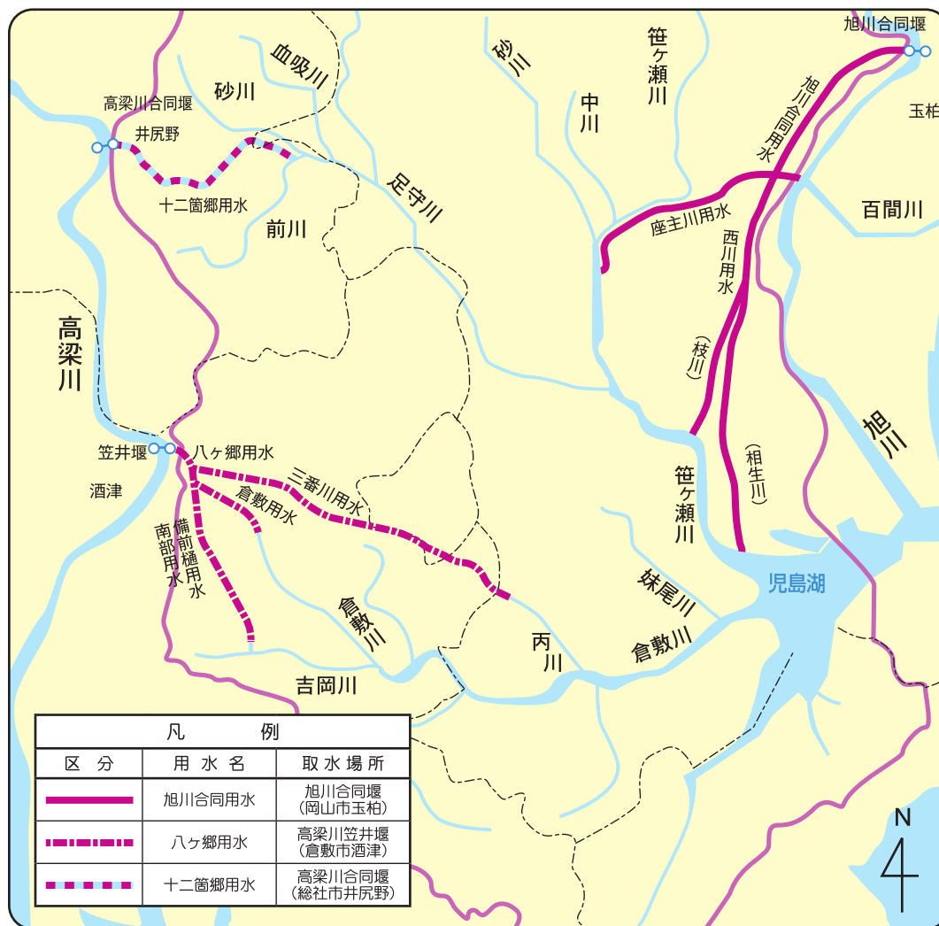
農業用水の再利用の主要水路系統図
