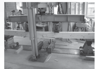
強度試験機による木材性能試験
