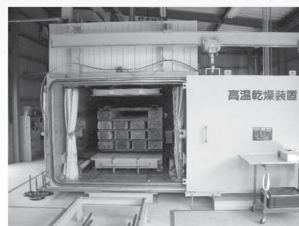
人工乾燥装置による木材乾燥
