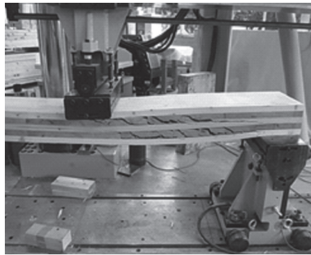
ヒノキを表層に使用したCLTの曲げ試験
