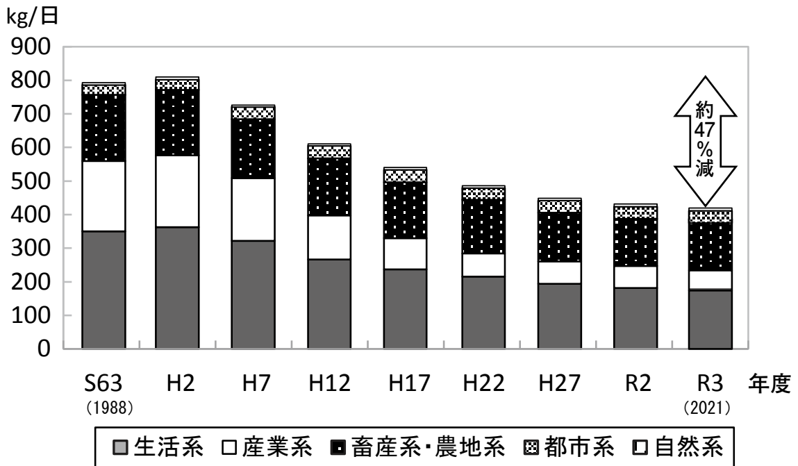
図2-19 全りん排出汚濁負荷量の削減状況
