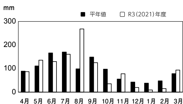
図 1-6 岡山市の降水量 (mm)
