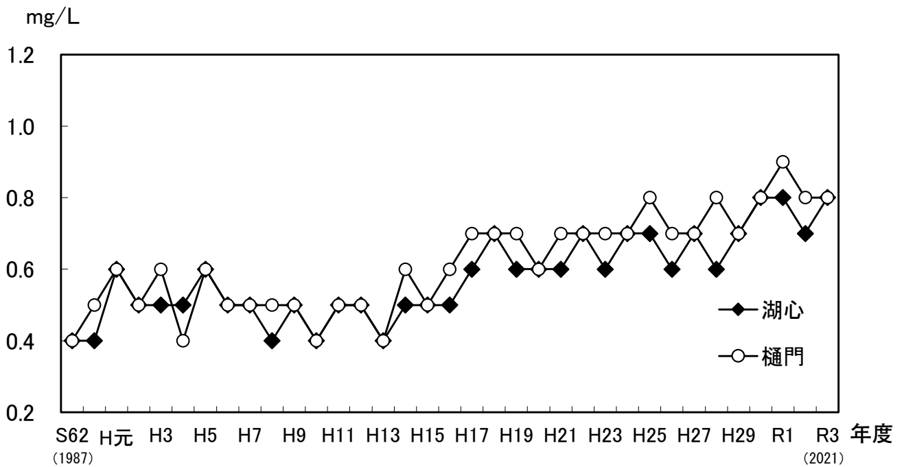
図2-6 児島湖の透明度（年平均値）の推移
