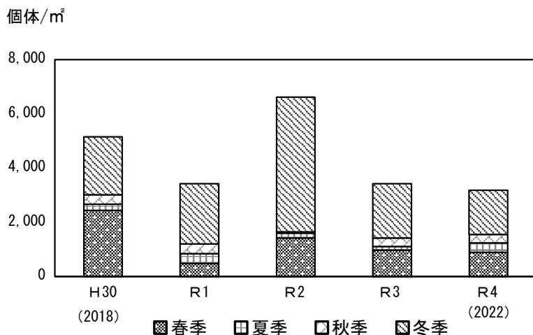
図 1-9 湖南におけるユスリカ幼虫個体数の推移
