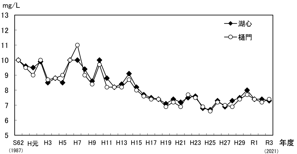
図 2-3 児島湖のCOD (年平均値)の推移
