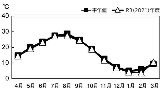
図 1-5 岡山市の気温 (℃)
