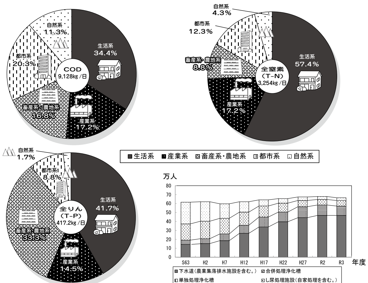
図2-20 COD、全窒素、全りんの発生源別割合 (令和3 (2021) 年度) 及び生活排水処理人口の推移
