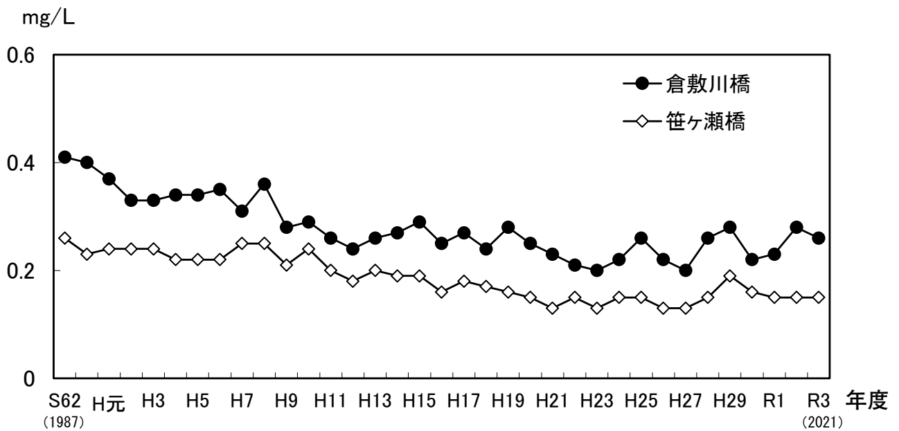
図 2-13 流入河川の全りん（年平均値）の推移
