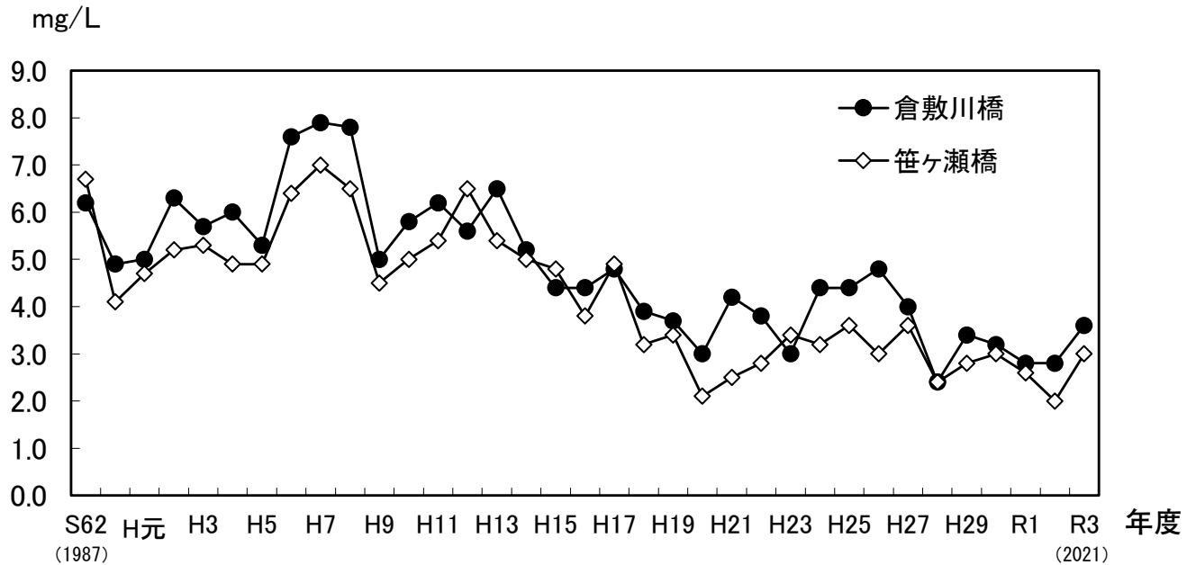
図2-10 流入河川のBOD (75%値)の推移
