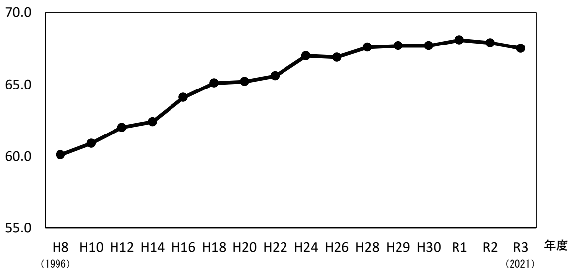
図 1-2 児島湖流域内の人口の推移
