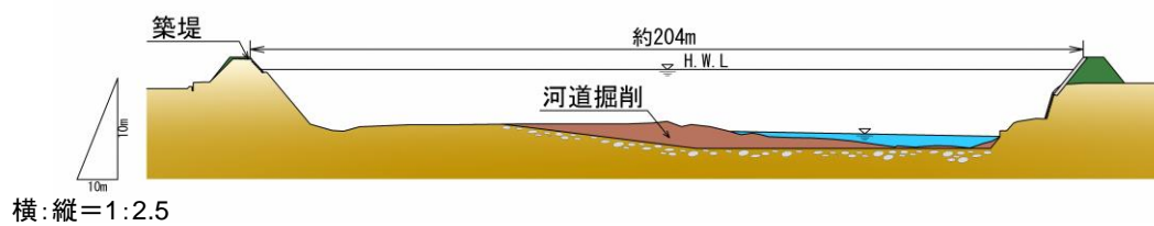
图 3-1-5(4) 旭川本川施行区間（建部町小倉～建部町福渡地区）横断面图（36K800）
