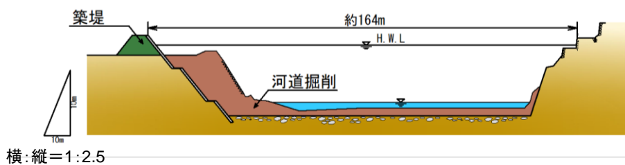
图 3-1-5(2) 旭川本川施行区間（御津国ヶ原地区）横断面图（26k800）
