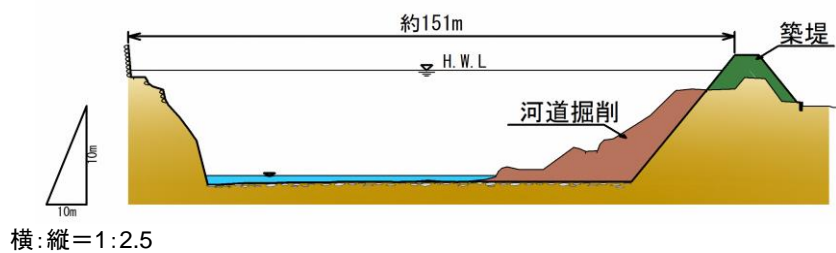
图 3-1-5(1) 旭川本川施行区間（中牧地区）横断面图（22K800）
