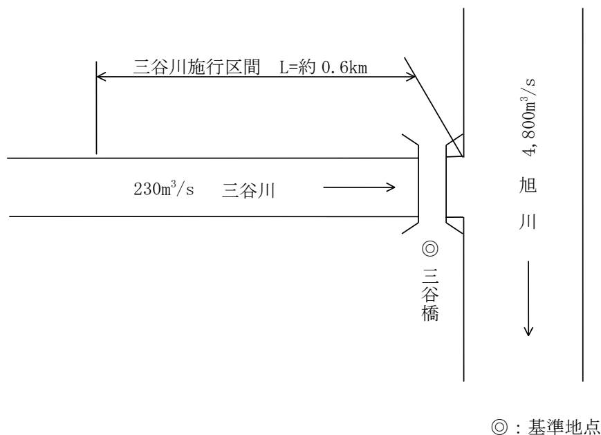
図 3-1-6 三谷川施行区間 整備計画目標流量配分図
