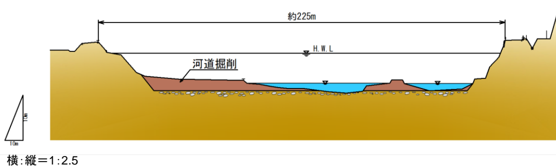
图 3-1-5(3) 旭川本川施行区間（御津宇垣地区）横断面图（28K800）
