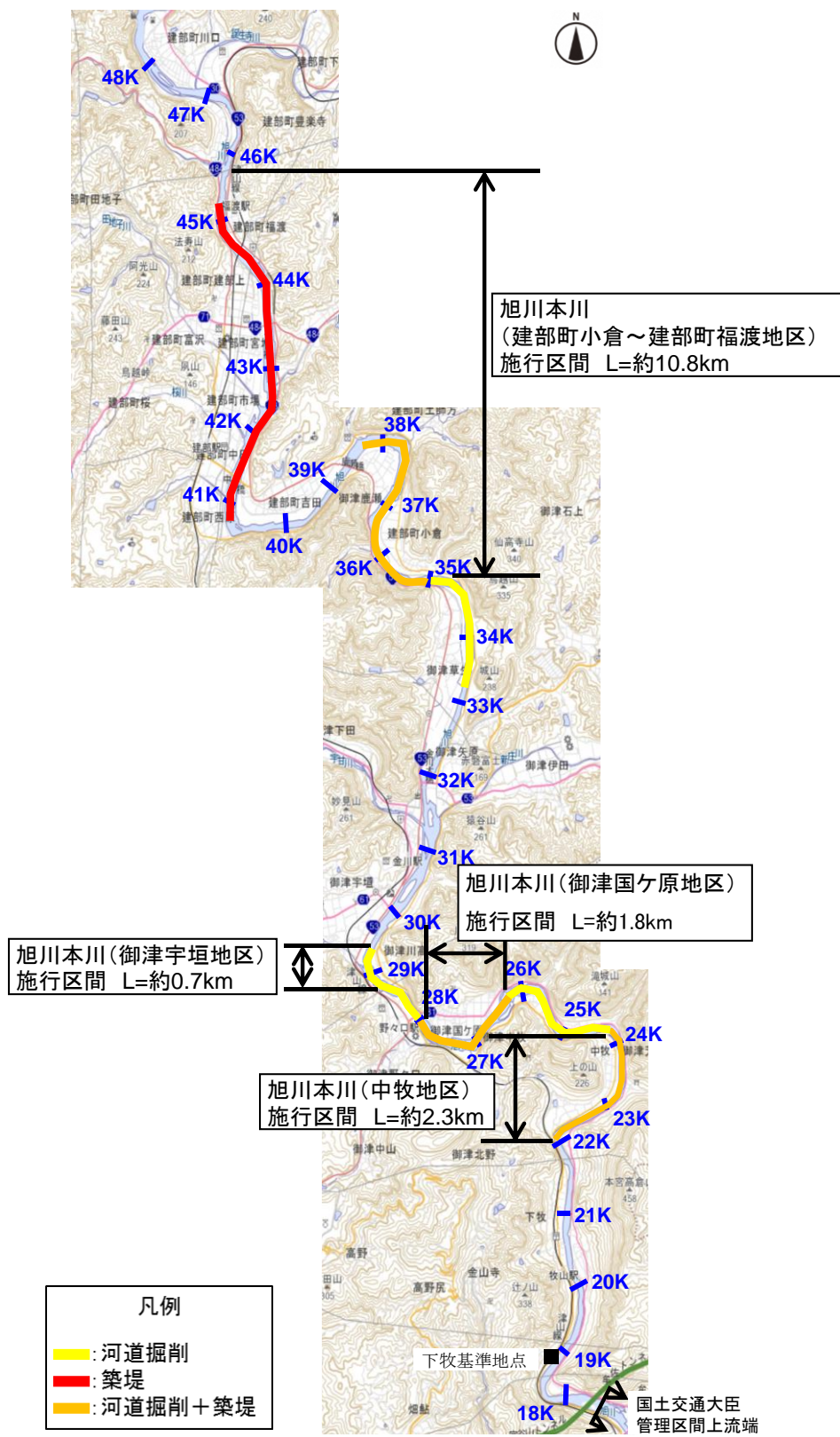
図 3-1-3 旭川本川施行区間 河川工事位置図
