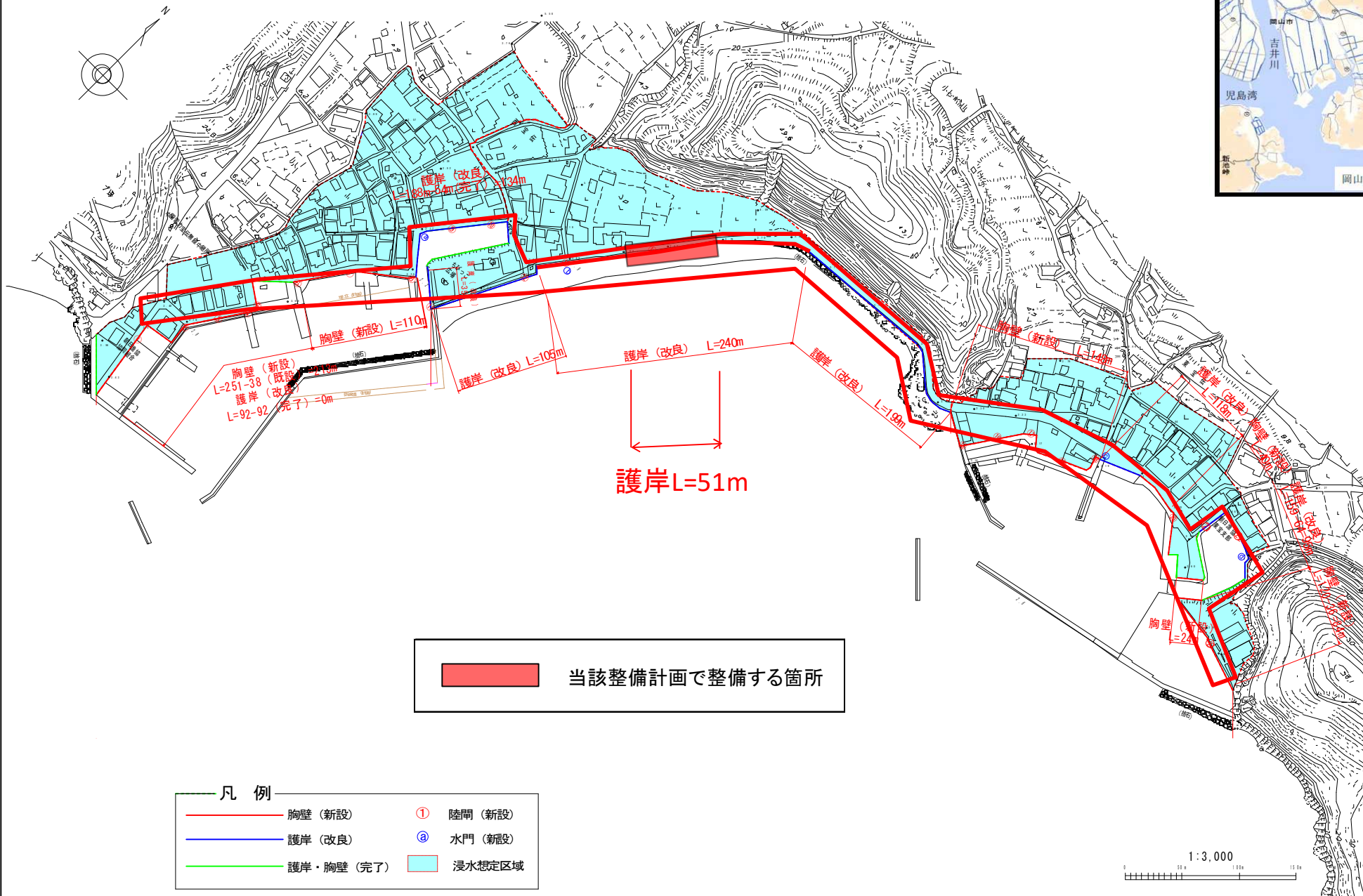
朝日漁港海岸平面図
