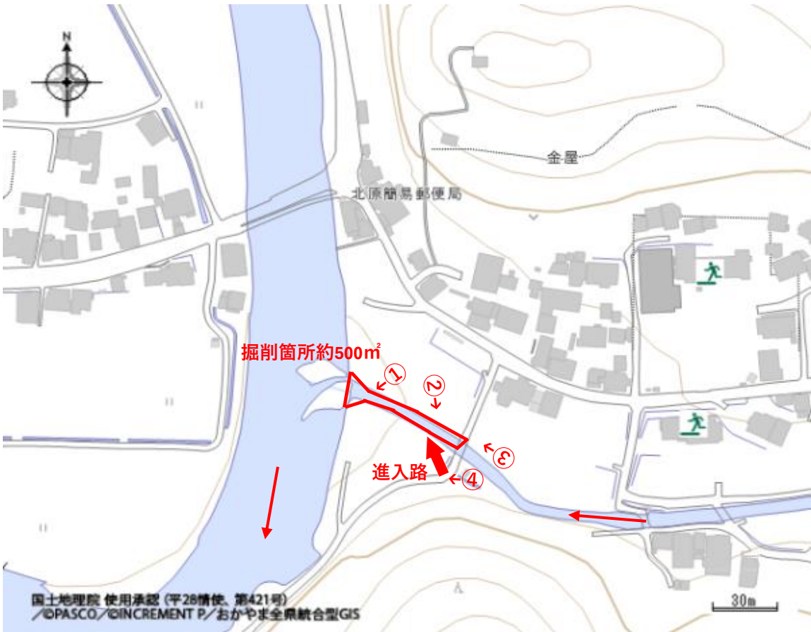
《平面図》
