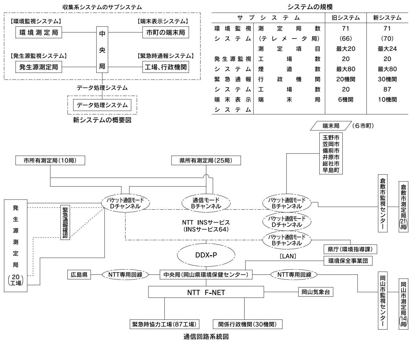
図2 - 7：大気汚染監視システムの概要
