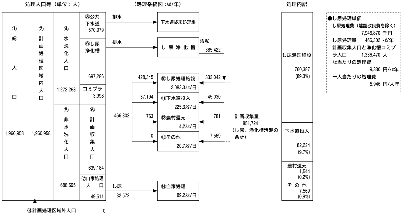
図5 - 3 : し尿処理の状況 (平成9年度実績)
