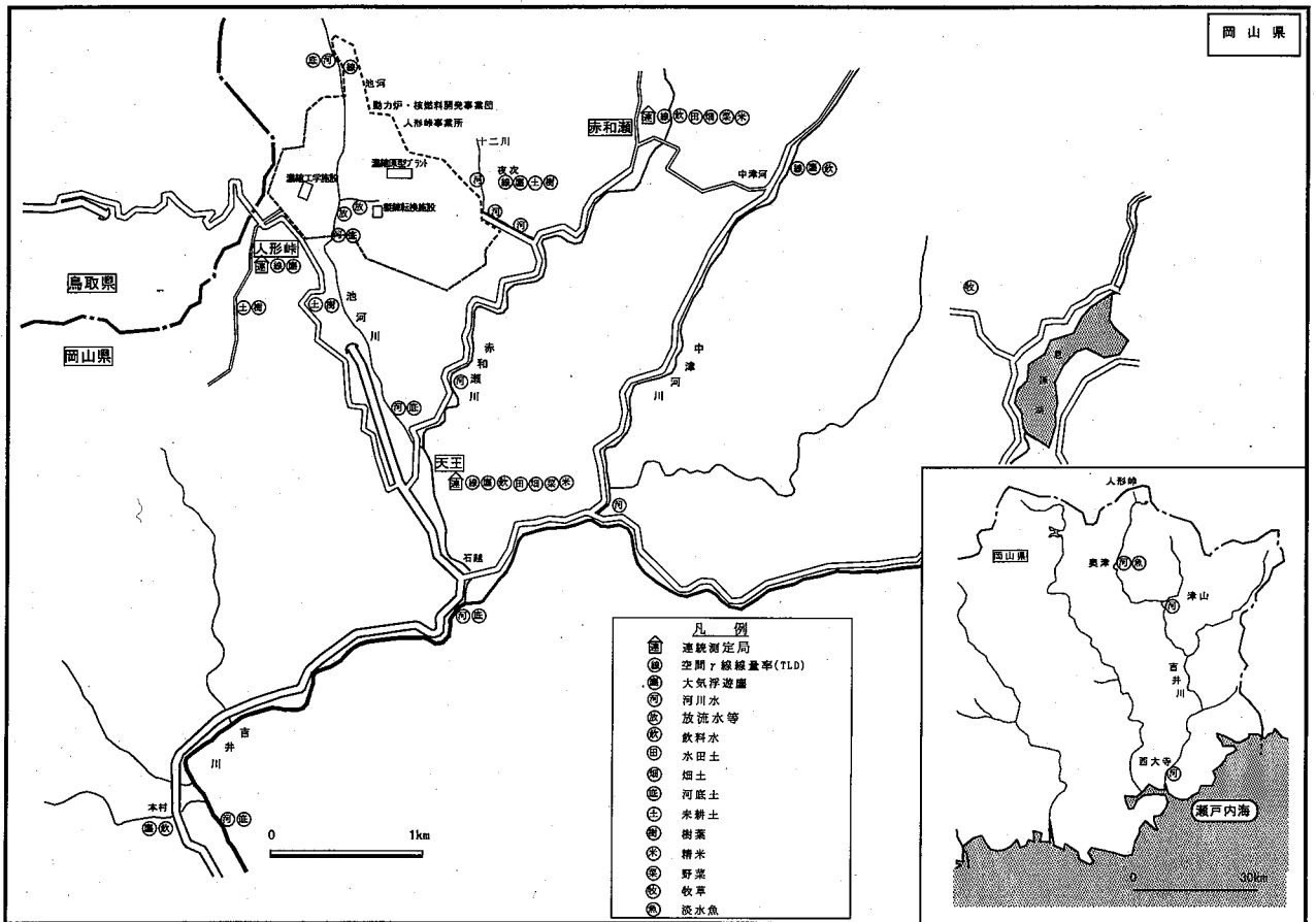
図2-7-1：人形峠事業所に係る環境放射線等監視測定地点
