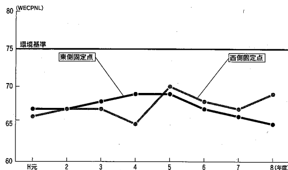
図2-3-6：航空機騒音の環境基準達成状況
