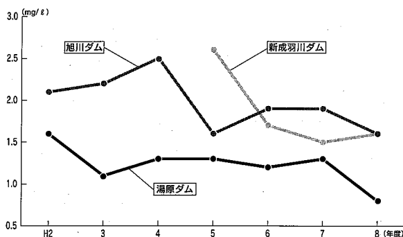
図2-2-5：ダム湖水質経年変化(BOD：75%値)
