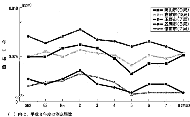
図2-1-1：二酸化硫黄濃度の年平均値の推移
