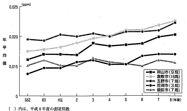
図2-1-3：二酸化窒素濃度の年平均値の推移(一般局・地域別)
