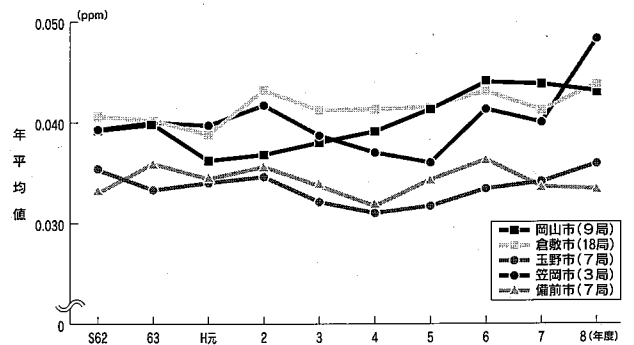
図2-1-6：浮遊粒子状物質濃度の年平均値の推移(一般局・地域別)
