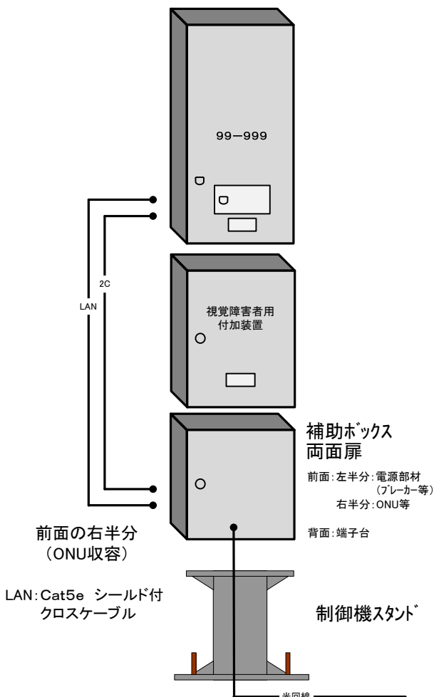
＜ 補助ボックス内部設置図 ＞
