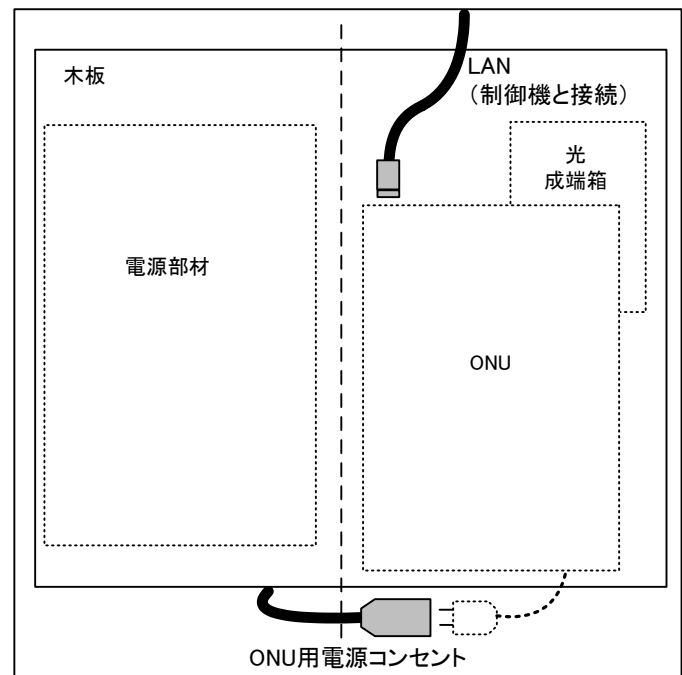
＜ 補助ボックス内部設置図 ＞
