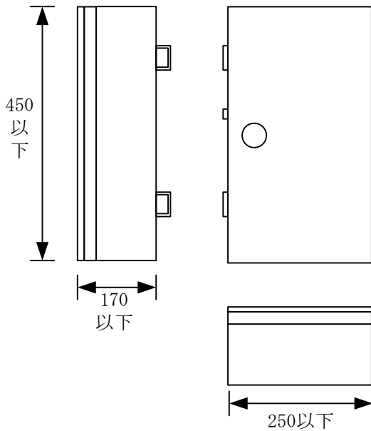
ONU收容箱
