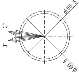
アルミポール断面図 (ギザ付き)
