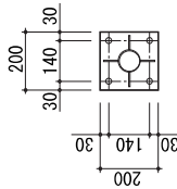
柱脚部の詳細図 S = 1 / 2 0
