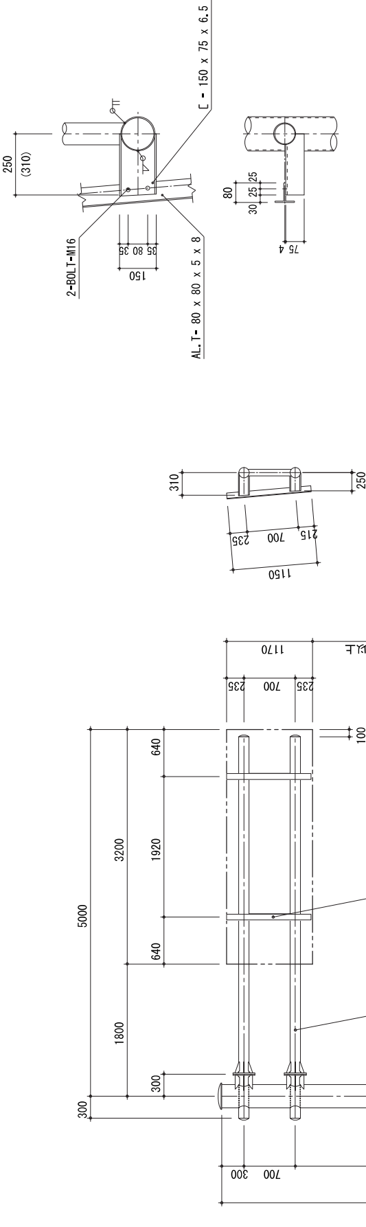
板取付金具詳細図 S = 1 / 1 5
